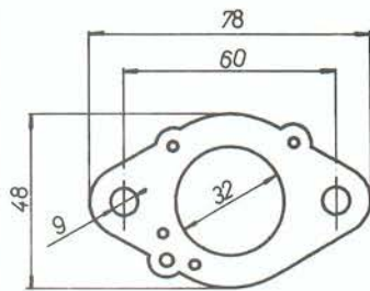
7237 32 PDSIT-2-4-7
