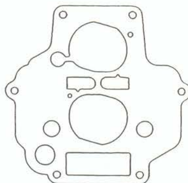
8097 32/34 DMTE Fiat Uno CS - Duna 70
