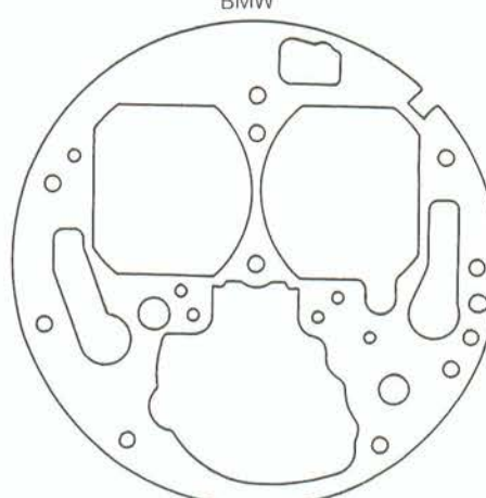
7942 35/40 INAT BMW - Opel - Mercedes
