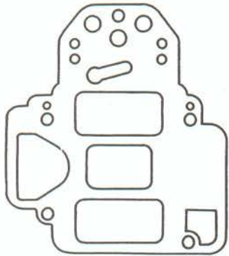
7118 40 DCOE
