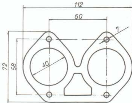
7231 Fulvia 2 C
