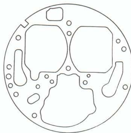
7664 35/40 INAT BMW
