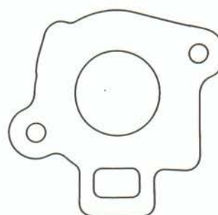
7851 Varajet Ford Escort
