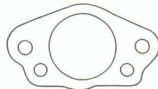
8018 S.U. HS 6 Austin - Innocenti - Jaguar MG-Morris - Rover Triumph - Volvo
