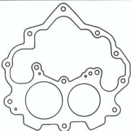
7340 35/40 INAT
