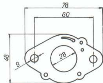
7251 28 PDSIT-7
