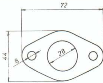
7310 Volkswagen 1200
