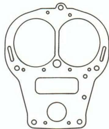
7263 Ford 17 M
