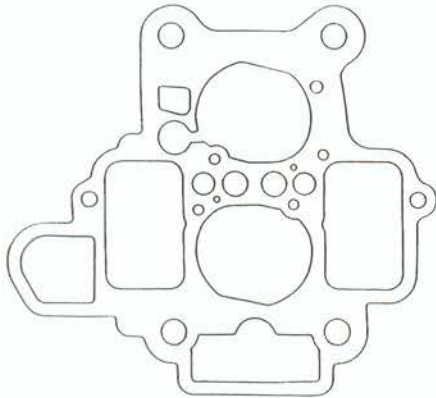
7970 32 DRT Renault R9 - R11
