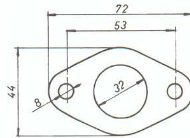
7312 Volkswagen 1500
