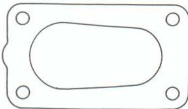
7630 Opel Commodore 2,5
