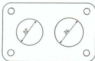
8060 32/35 TCICA Citroën BX 14 E
