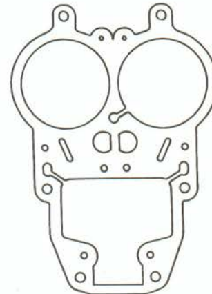
7713 34 TEIE
