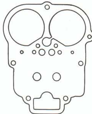
7757 ZAZ - ZIGULI - LADA
