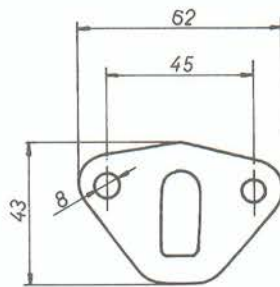
7313 Simca 1000 - 1300 - 1500
