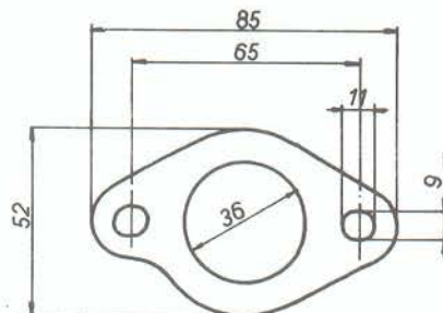
7270 Simca 1500
