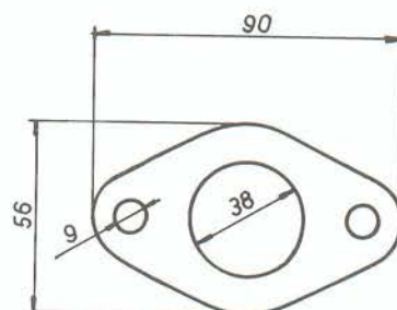
7305 BMW - Opel
