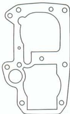
7859 32 IF Renault R5 GTL - R9
