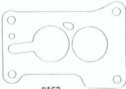
8162 Toyota Carina 1,8 Celica 2,0-Corona 2,0 Aisan
