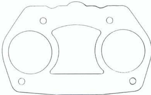
8201 Fiat 124 Abarth 44 IDF
