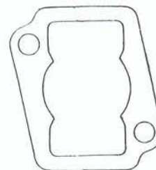
8263 Lancia Dedra 1,6 Fiat Tipo-Tempra Monoiniettore Weber
