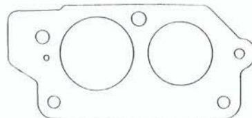
8189 Hundai Poni 1,3 L - GLS - 1,5 GLS Aisan
