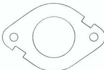
8264 Alfa 33 40 DRLA-40 IDF
