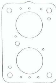
8150 Renault R19 32/32 TLDR
