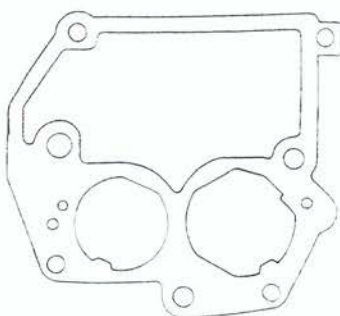
8273 Volksw. Golf-Mercedes 2 EE Ecotronic
