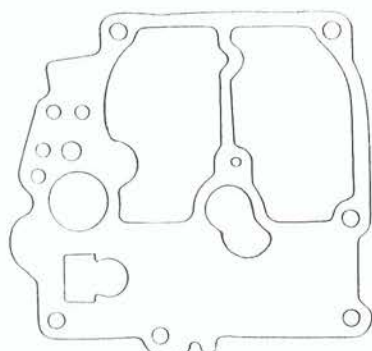
8160 Toyota Carina 1,8 Celica 2,0-Corona 2,0 Aisan
