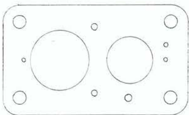
8259 Lada Niva 28/32 DGR
